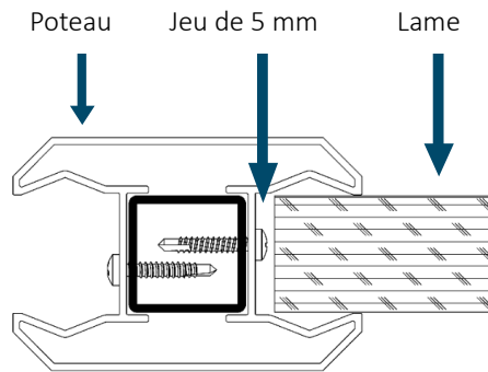
vue de dessus du poteau
