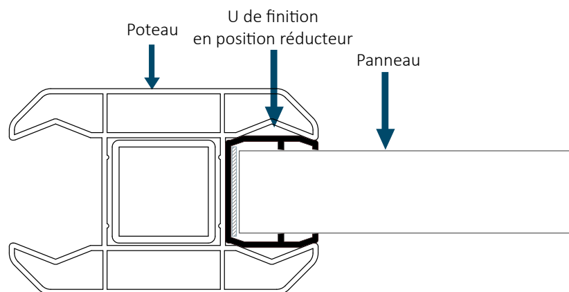
vue de dessus du poteau
